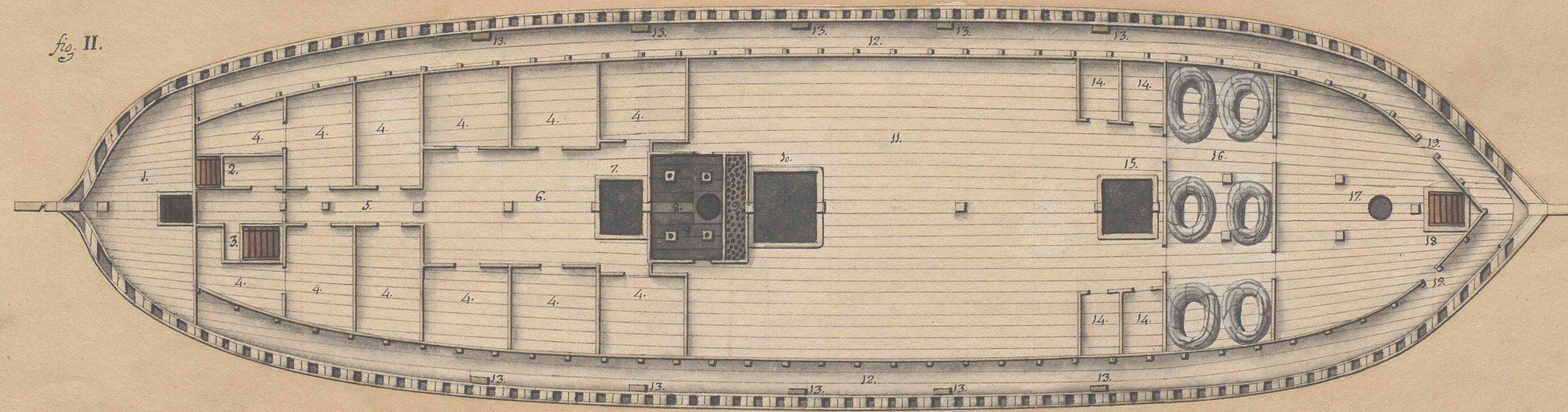
Fig. I. Tercera seccion de la Bodega de un Navio de 74 cañ. es (que pasa por la lin. E, F, de las Lam. as III, y IV,) y manifiesta la colocacion de la 3. a andana de Piperia, Cables, &c.
