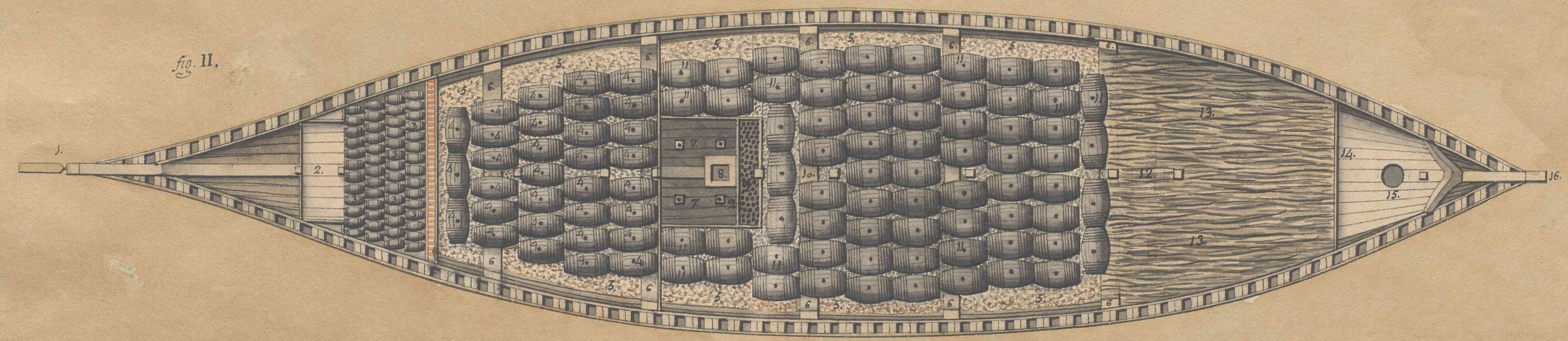
Fig. I. Primera seccion horizontal de la Bodega de un Navio de 74 cañ. (que pasa por la linea A, B, lam. III, y IV.) y representa la colocacion del Sustrate de fierro en cañ. baxos, y lingotes.
