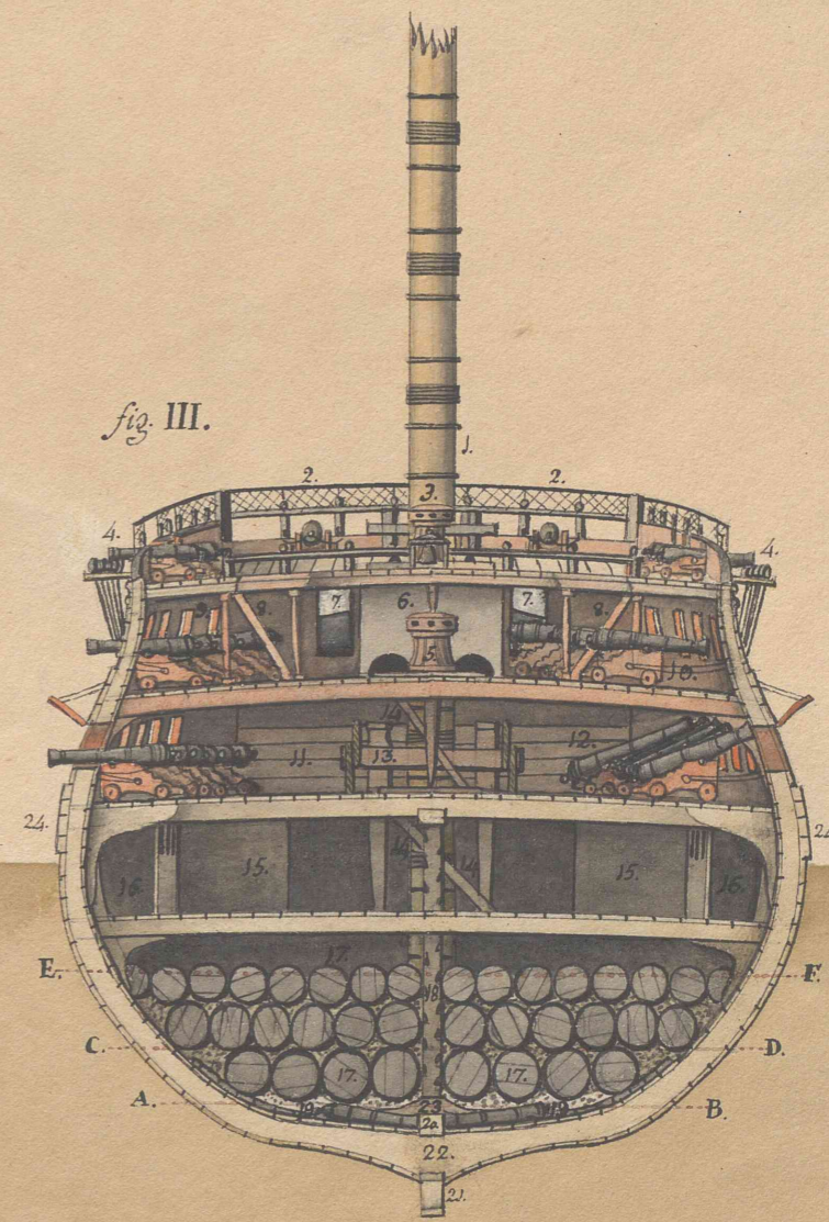
Fig. III. Vista interior del mismo, considerado por una sección vertical por la Quadera maestra.
