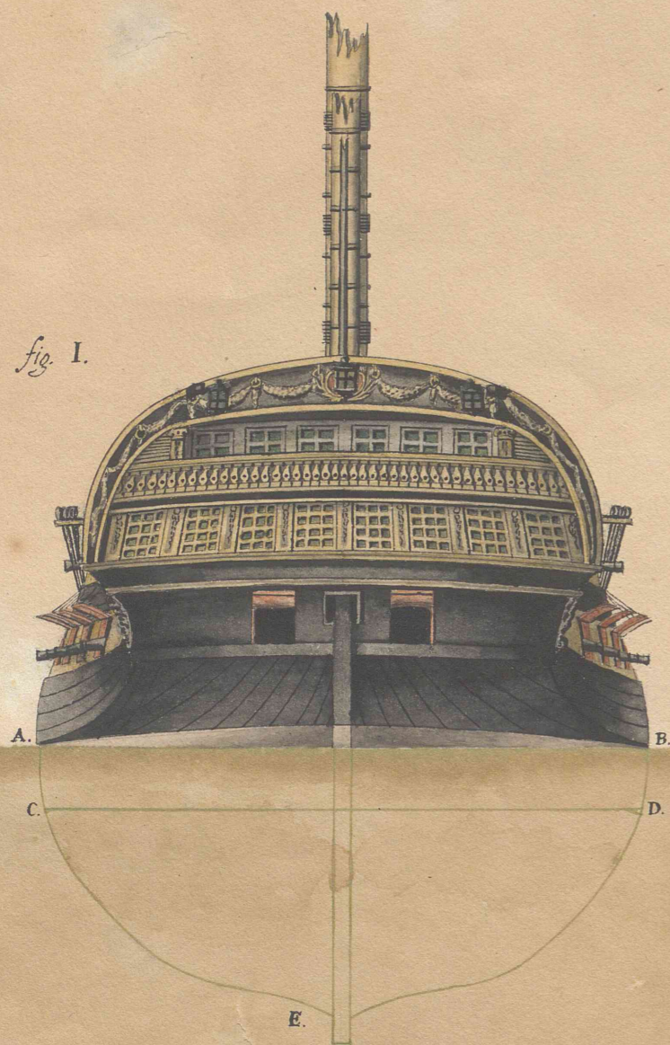
Fig. I. Navio de 74 cañones, visto por la Popa.
