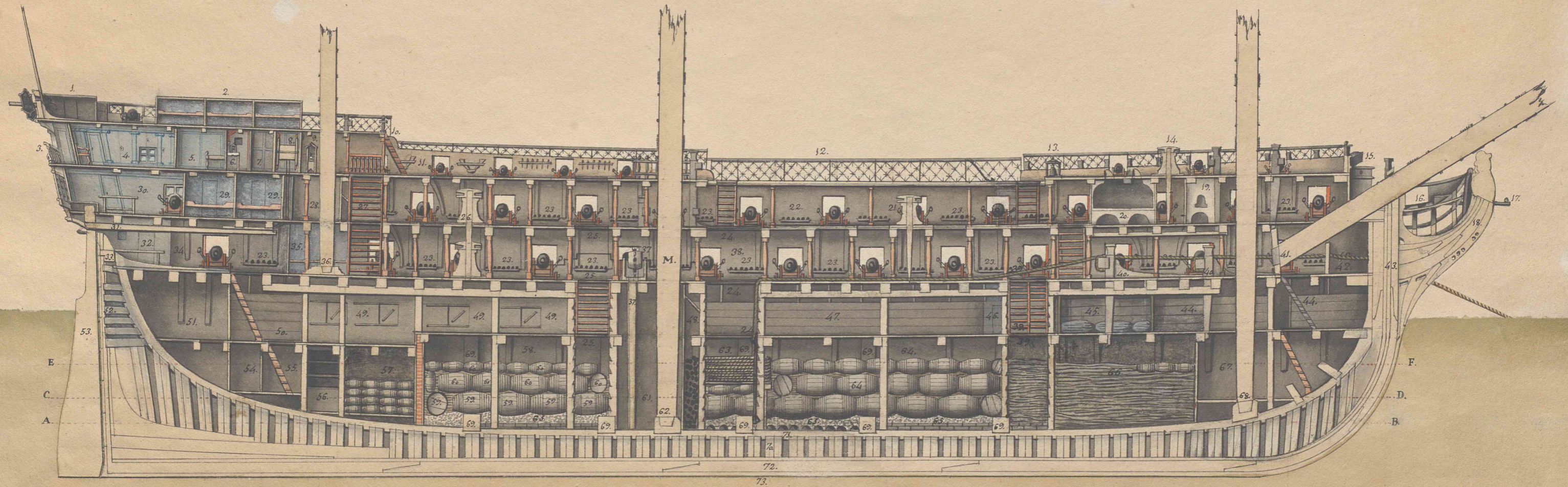
Vista interior de un Navio de 74 cañones, considerado por una seccion vertical de Popa à Proa, en el sentido de la Quilla.
