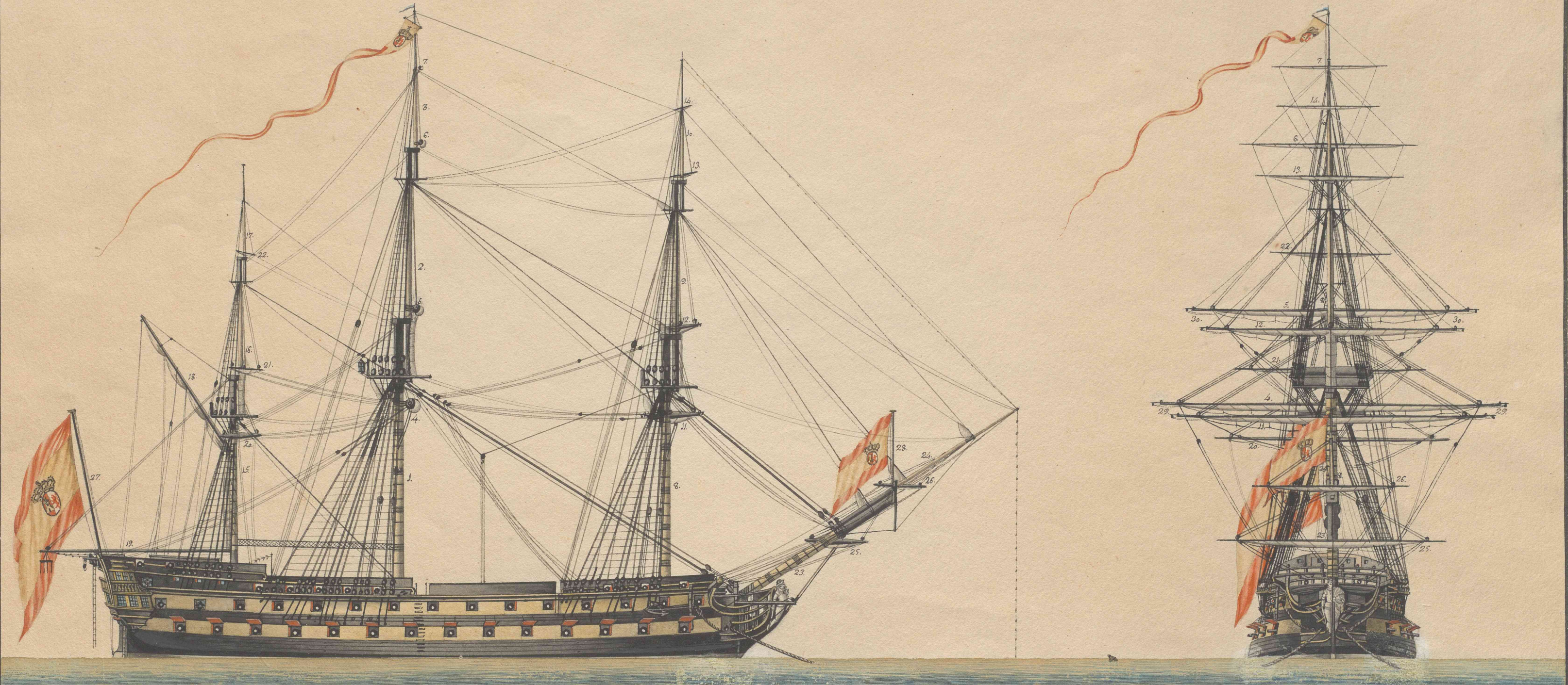
Navio de 74 cañones aparejado, visto en las dos posiciones de Proa, y de Costado, que manifiestan la proporción, y dimensiones de su Arboladura
