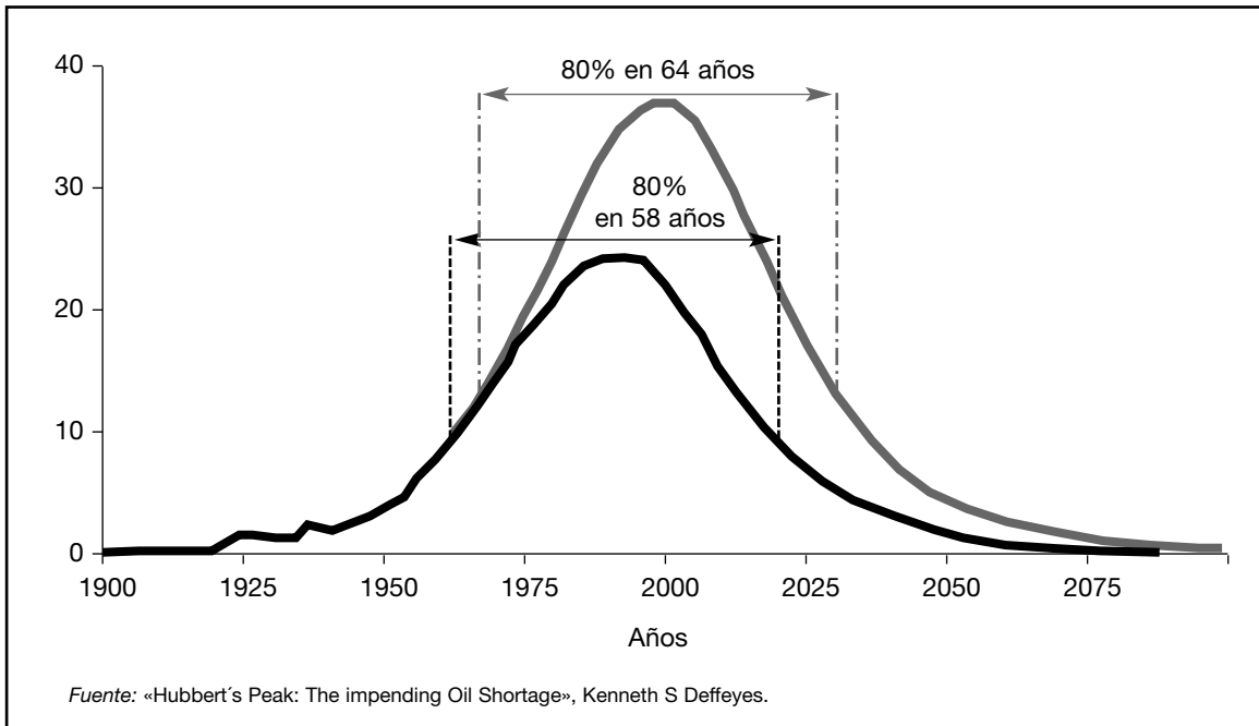
Figura 1. – Proyección de la producción mundial de petróleo realizada por Hubbert en 1971 y publicada en Scientific American.
