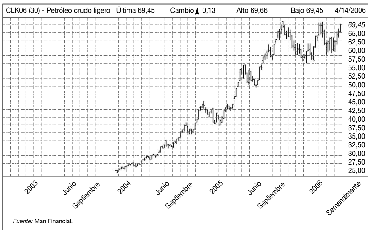
Figura 3. – Subida del precio del petróleo.
