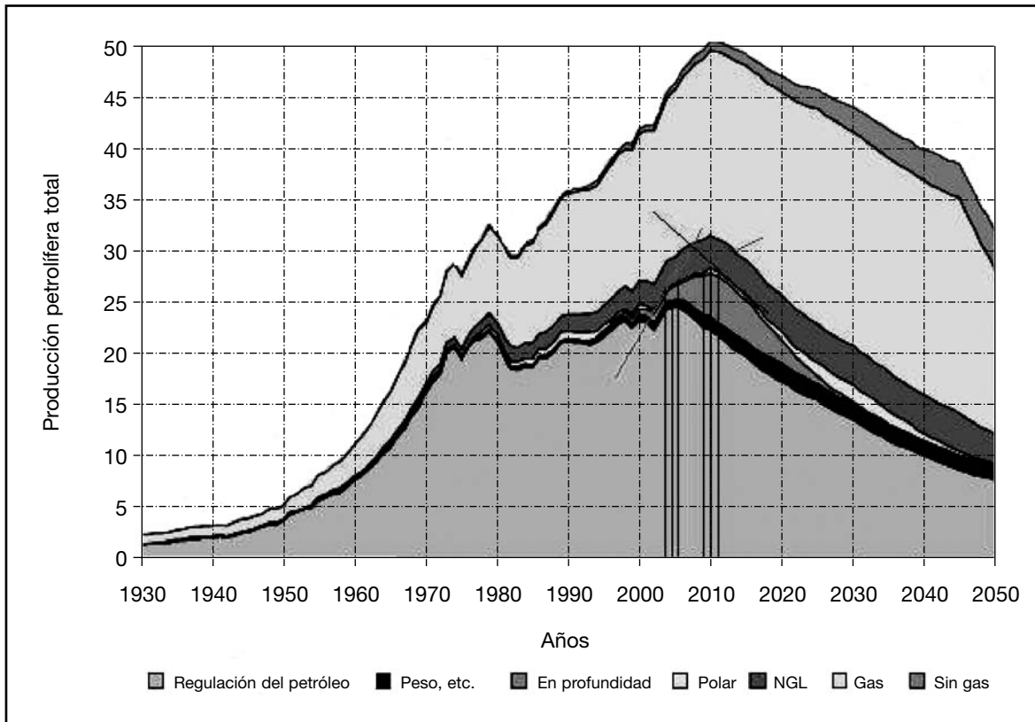
Figura 2. – Proyección de la producción del petróleo y el gas.
