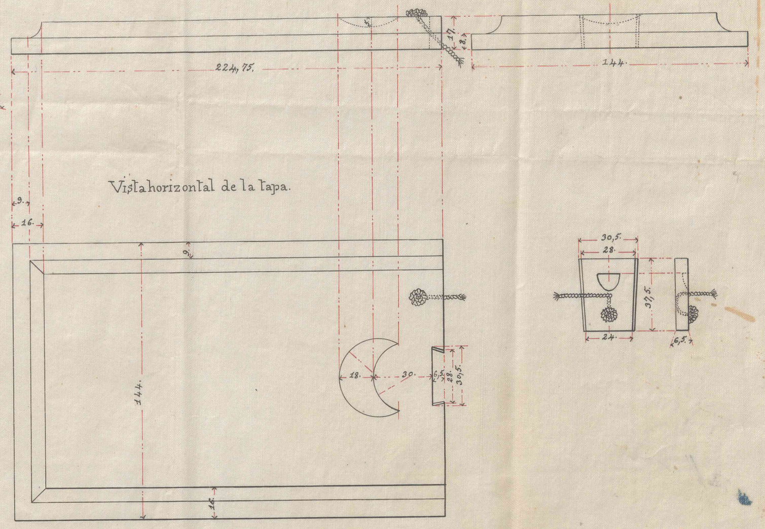
Caja para cabezas - portacebos del n.º 3.
