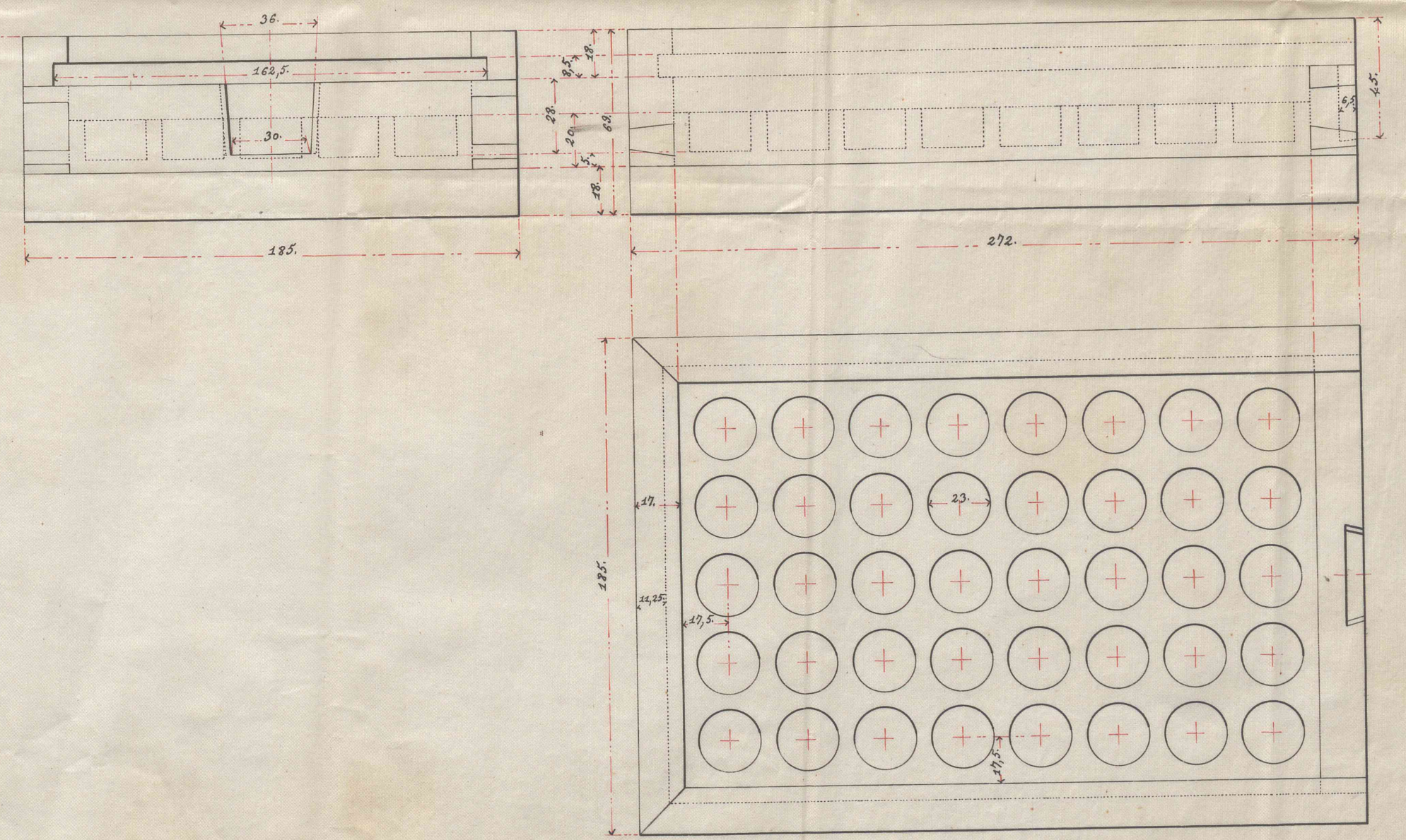
Caja para cabezas - portacebos del n.º 3.
