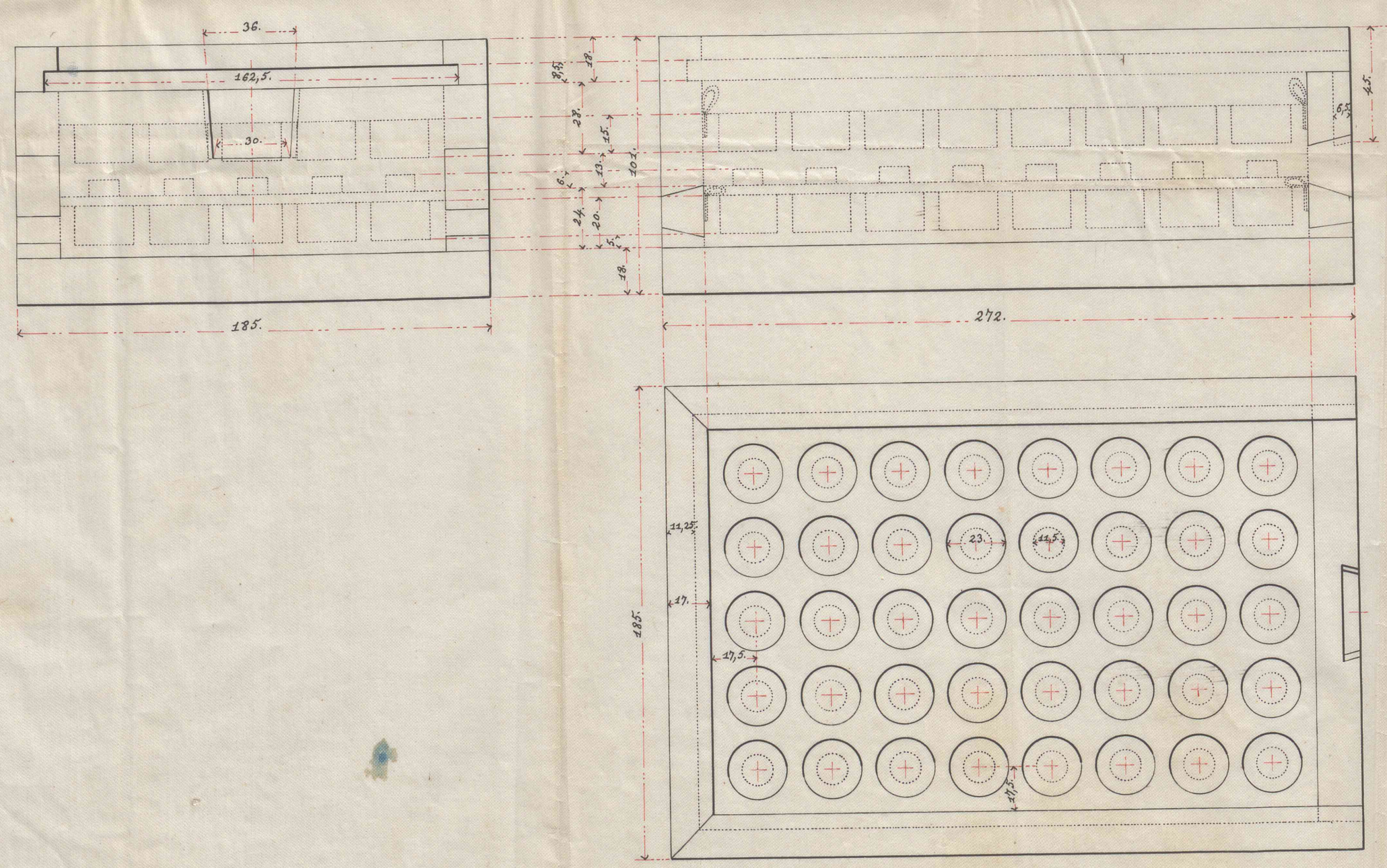
Doble caja para cabezas - portacebos del n.º 3.
