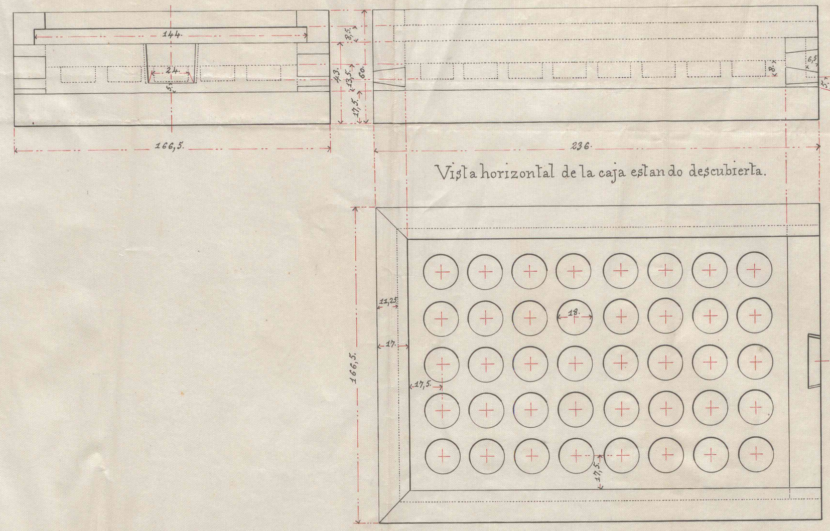
Caja para cabezas - portacebos del n.º 2.
