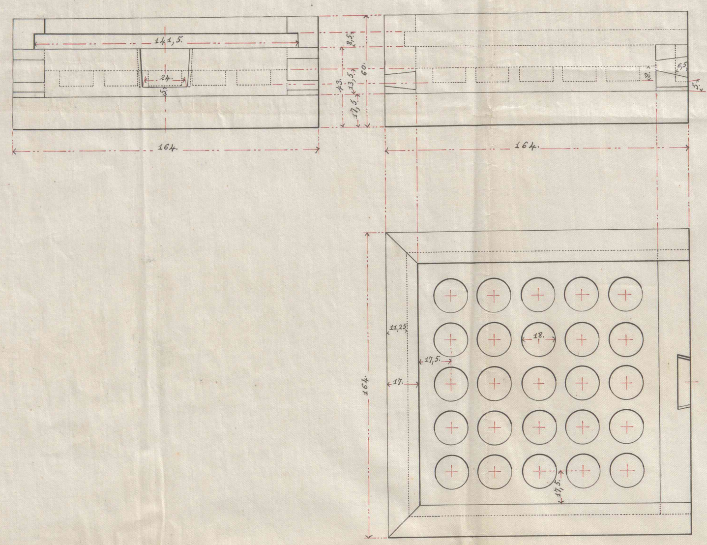
Caja para cabezas - portacebos del n.º 1.
