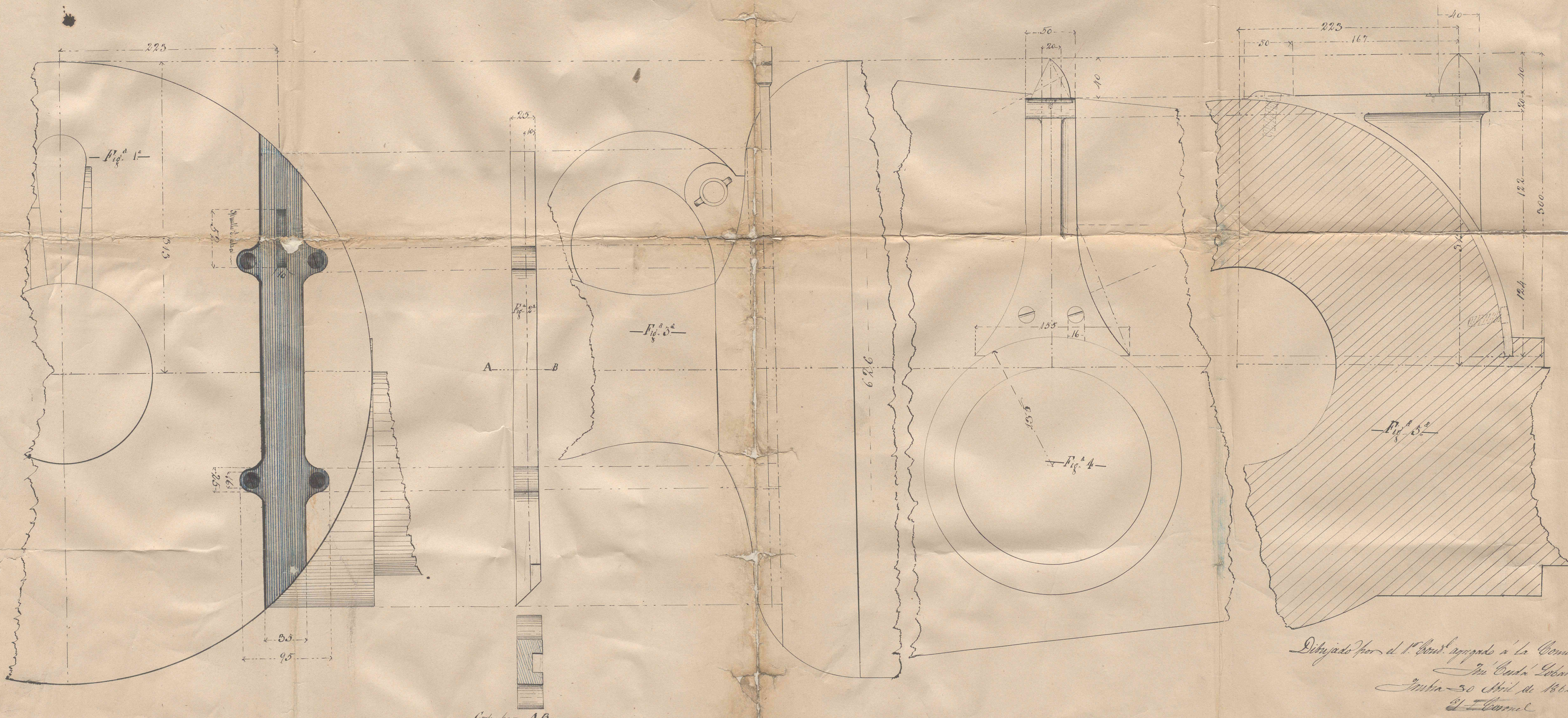
- Corte por A B -
