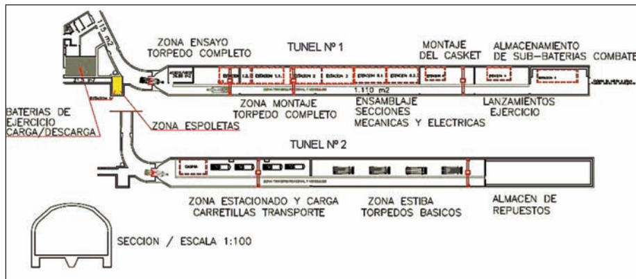
Disposición de uso prevista para los túneles número 1 y número 2.
