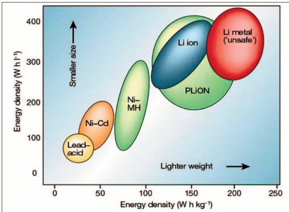
Densidad energética de los diversos materiales empleados en la elaboración de baterías. (Fuente: www.wikipedia.org )
