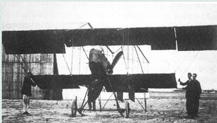
El BCD 1 «Cangrejo», de los primeros aviones españoles que volaron con regularidad. Cuatro Vientos, Madrid, 1912
